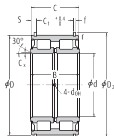
S pojistným kroužkem
