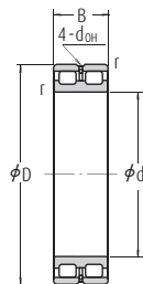
Volné ložisko RSF
